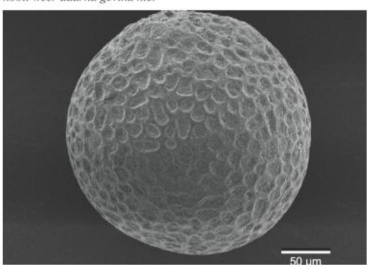
'n Foto van die skaars feetjiegarnaal se eiertjie, geneem deur 'n skandeer elektronmikroskoop. Elke eiertjie wat deur die spesies in die Branchiopoda groep gelê word se morfologie is uniek tot elke spesie. Hulle kan dus gebruik word om spesies uit te ken deur droë grondmonsters onder die mikroskoop te ontleed. Hierdie piepklein (± 240 µm) eiertjie verbreek onder enige druk sterker as 1 Newton-krag.
